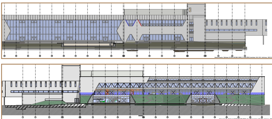
A velencei sportuszoda homlokzatának terve a Béke utca felőli (alul) és a Tó felőli oldalról
