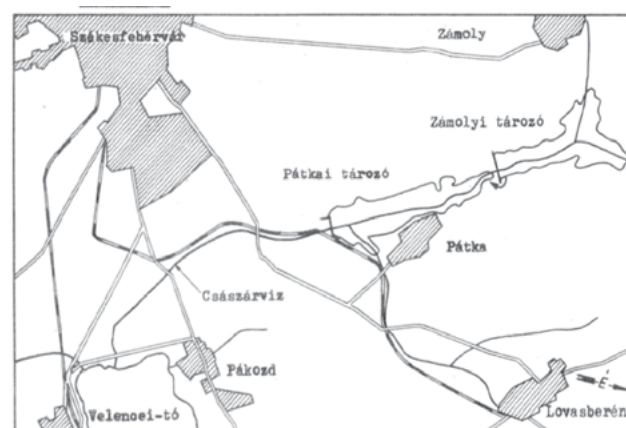
III.8. ábra: A Pátkai és Zámolyi tározók válsatos helyszínrajza
