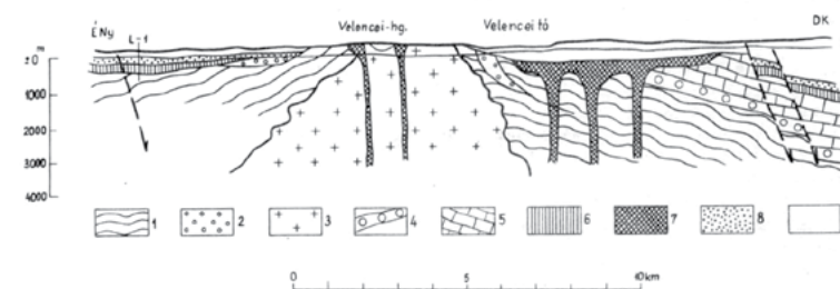
II.17. ábra: A Velencei-hegység és környéke szerkezeti szelvénye /Wein Gy. 1971/. 1. ópaleozoós kristályos kőzetek, 2. alsókarbon konglomerátum és agyagpala, 3. felsőkarbon gránit, 4. perm konglomerátum és homokkő, 5. mezozoós, főként karbonátos kőzetek, 6. paleogén rétegek, 7. felsőecén andezit, 8. miocén homokos-agyagos rétegek, 9. pliocén és kvartár homokos-agyagos rétegek.
