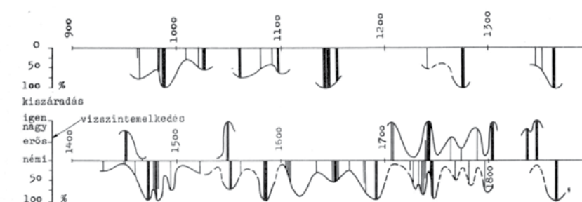
II.18. ábra: A Velencei-tó vízszintingadozásai i.u. 900-tól 1900-ig, egykori feljegyzések és Réthly A. nyomán.
