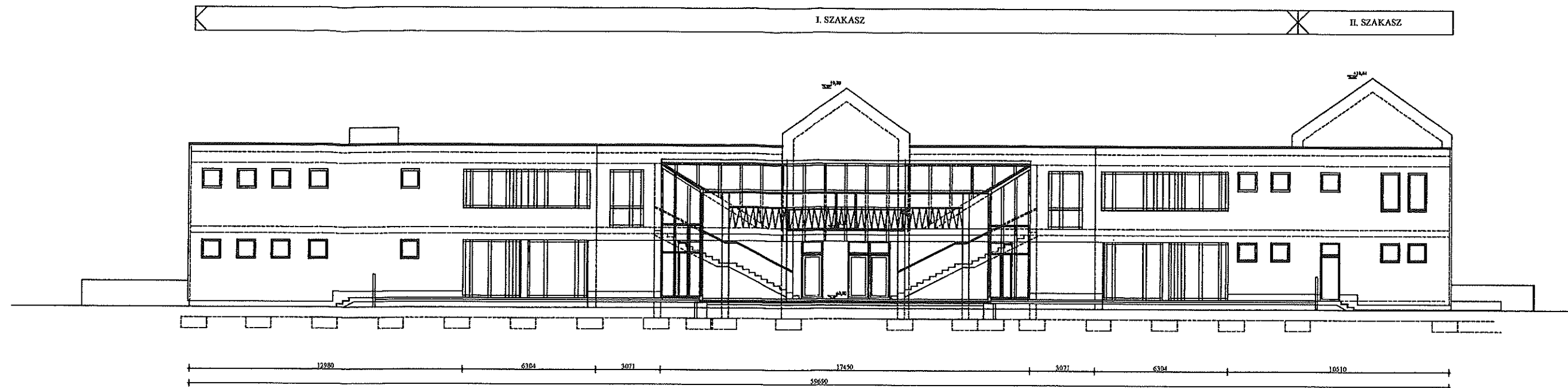
B - B METSZET M 1 : 200
